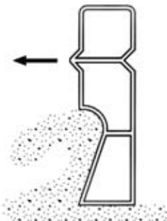
PERFIL DEL REGLE (ESPECIAL PARA SUPERFICIES DE HORMIGÓN)
