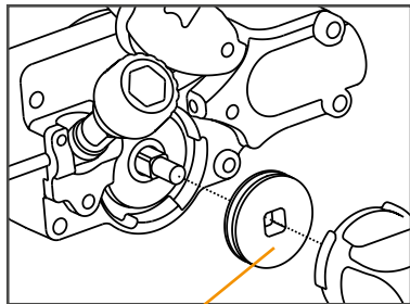
ROLDANA
